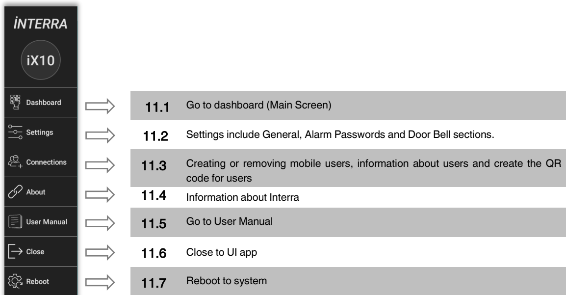
Fig. 53: Side Menu
