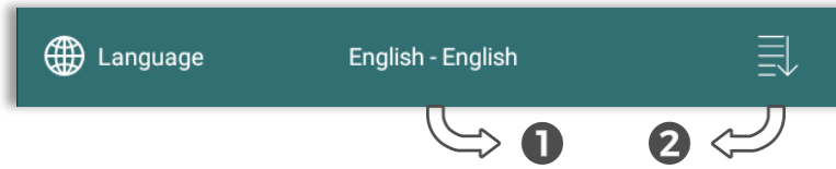
Fig. 67: Language Bar
